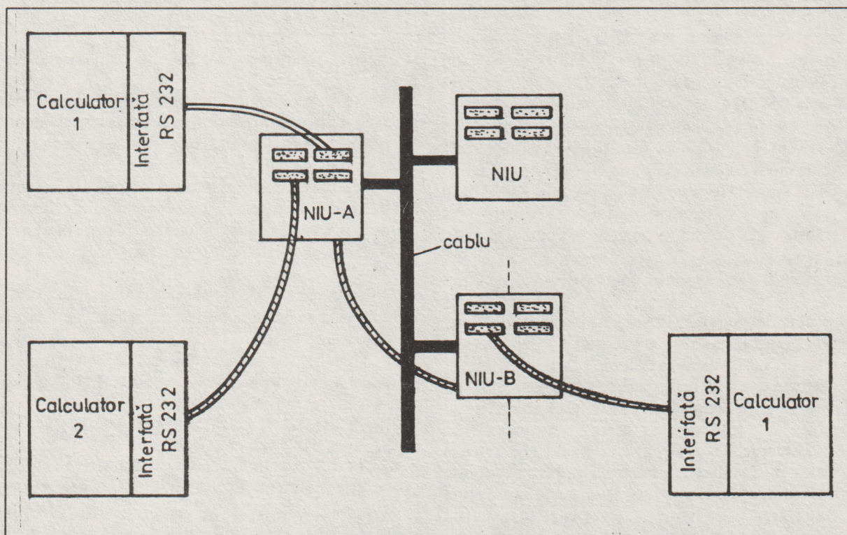
Figura 3. Retea locala de tip Ethernet (magistrala comuna)
