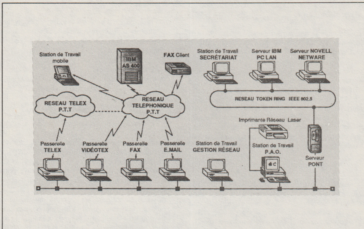
Figura 4. Rețea generală de transmisie de date
